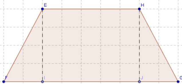
trapezio isoscele
