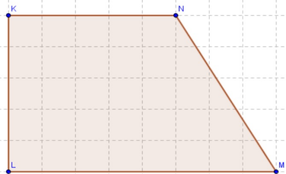
trapezio rettangolo
